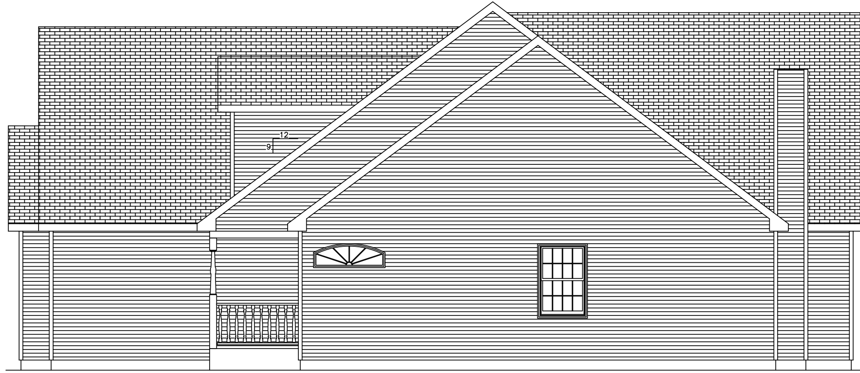
RIGHT ELEVATION
